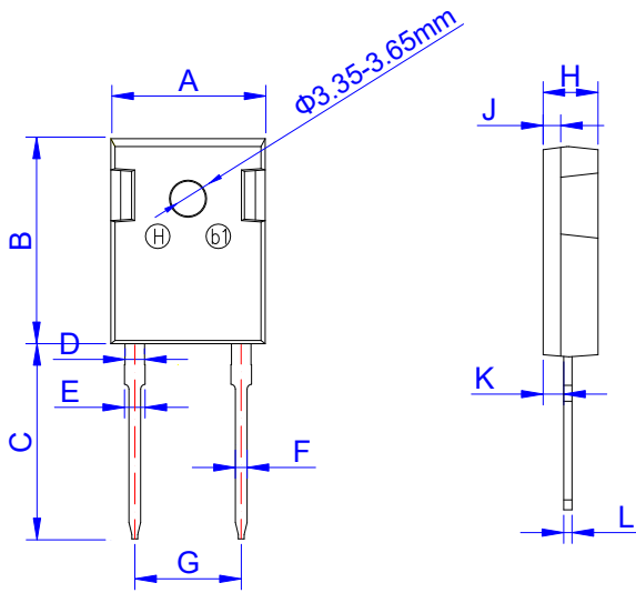
TO-247J-2L
